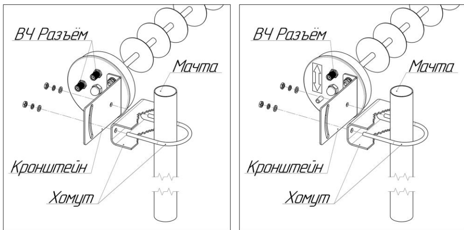
Схема 1 – Монтаж антенны на мачте
