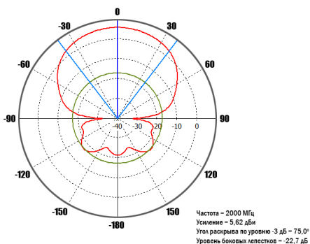
Коэффициент усиления антенны в рабочем диапазоне частот
