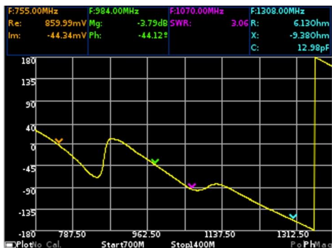
Рисунок 10.3 – График фазы
