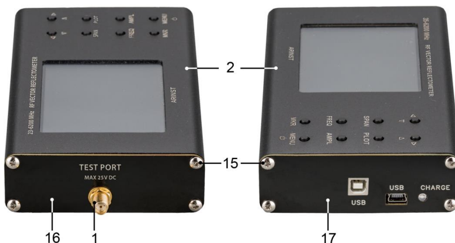
Рисунок 11.2 – Разборка корпуса прибора
