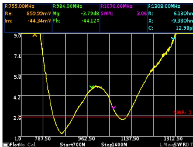
Рисунок 10.8 – График КСВН
