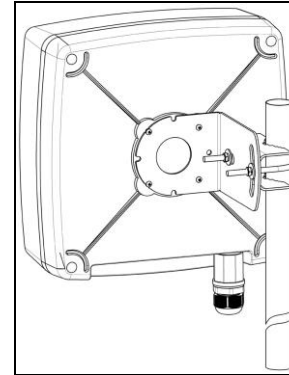
Рисунок 2 – Монтаж антенны
