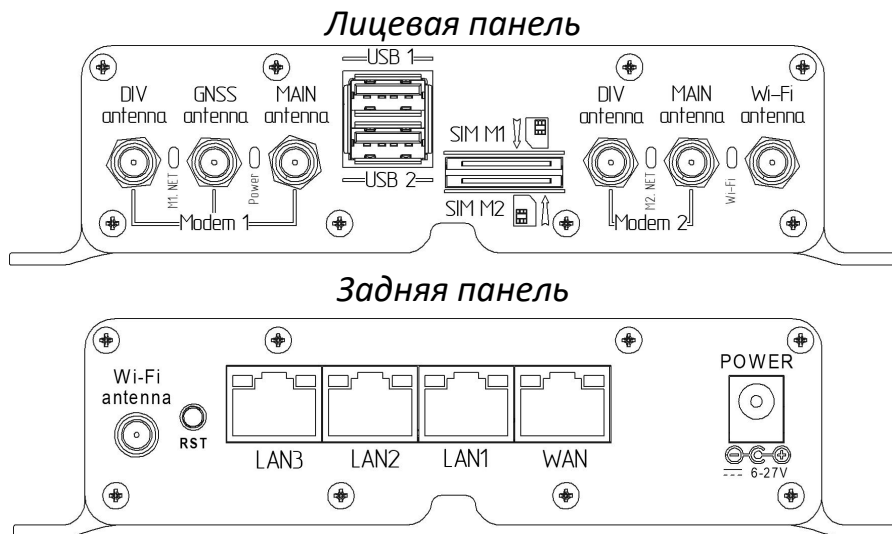
Схема 1 – Расположение индикаторов и портов устройства (для модификации с GPS)
