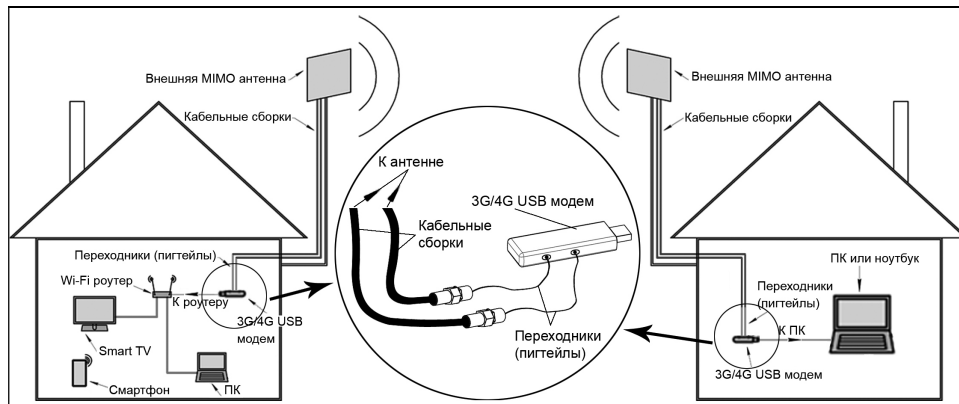
Схема 3- Примеры установки и подключения антенны к оборудованию
