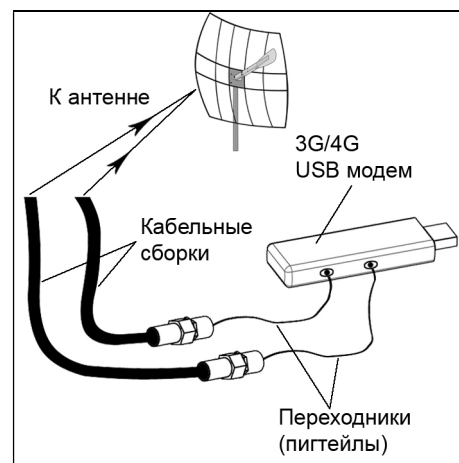
Схема 5 – Пример подключения 3G/4G USB модема к MIMO антенне
