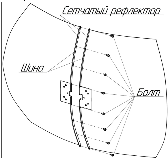
Схема 1 – Сборка сетчатого рефлектора антенны
