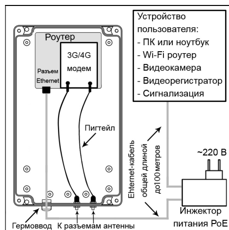
Схема 4 – Пример размещения оборудования в гермобоксе (приобретается отдельно)
