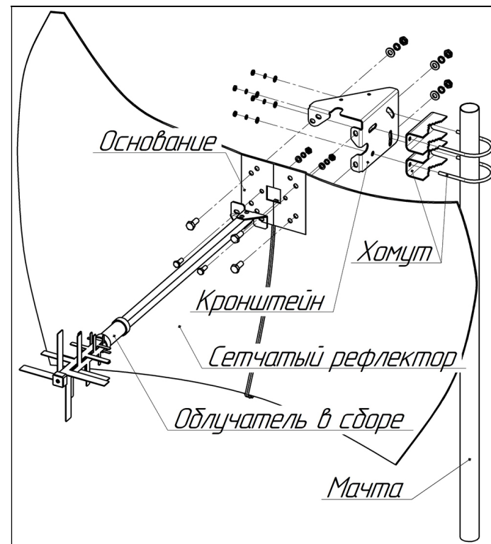
Схема 2 – Сборка сетчатой параболической антенны
