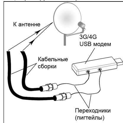
Схема 1 – пример подключения USB модема к ММО облучателю параболической антенны
